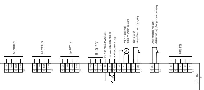
Схема подключения ШУПС-3 НВ (металл IP54)
